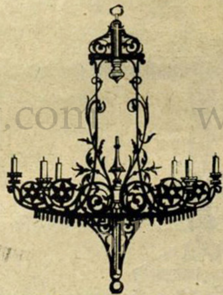
No. 537 Kronleuchter RM. —.25 48 cm hoch, 40 cm breit A. H. RM. 2.70 Dreherei RM. 4.20
